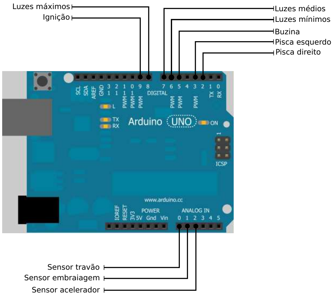
Figura 2.7: Esquema das portas utilizadas pelo Arduino responsável pela monitorização.
